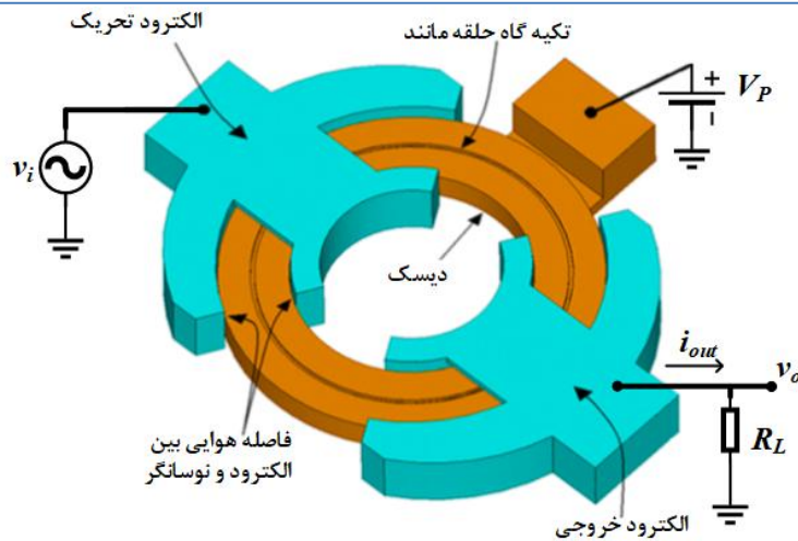
شکل (۱). نمای سه بعدی نوسانگر دیسک حالت محیطی با تکیه گاه حلقوی به همراه الکتروودهای تحریک، خروجی و بایاسیج [۶]
