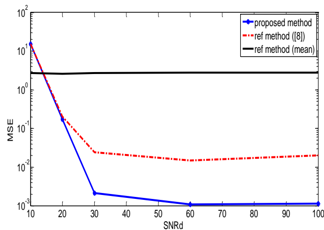
شکل (۶). مقایسه روش‌ها برای پیش‌کدینگ تحمیل صفر به ازای SNR_u = 0 و T_d = 1000
