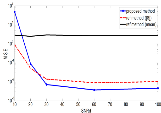
شکل (۵). مقایسه روش‌ها برای پیش‌کدینگ حداکثر نسبت به ازای SNR_u = 0 و T_d = 1000
