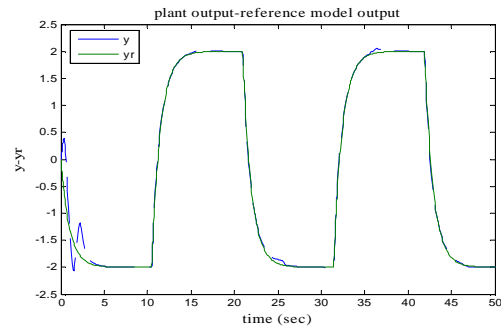
شکل ۱۱: خروجی فرایند و خروجی مدل مرجع
