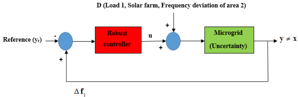
شکل ۴. ساختار ریزشبهه ناحیه یک با کنترل کننده پیشنهادی
