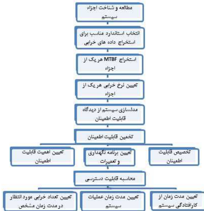
شکل ۱: روند تحلیل قابلیت اطمینان سیستم
